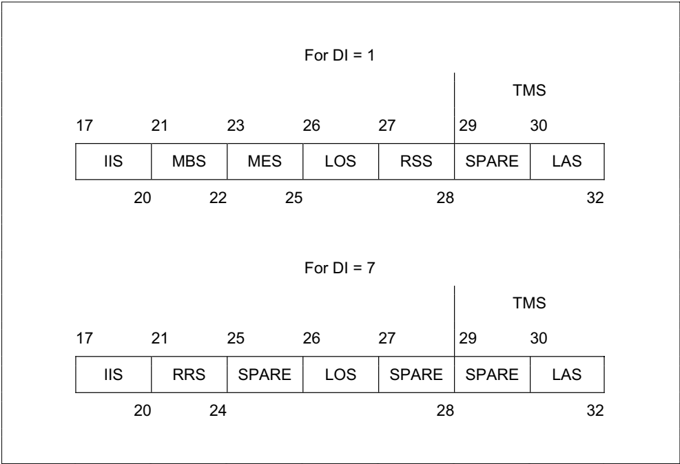
Rysunek 5-1. Struktura pola SD for di = 1 – dla di = 1; for di = 7 – dla di = 7
