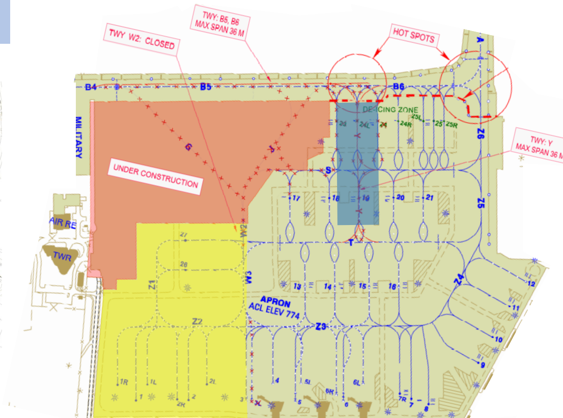
ETAP I FAZA II PLANOWANY
