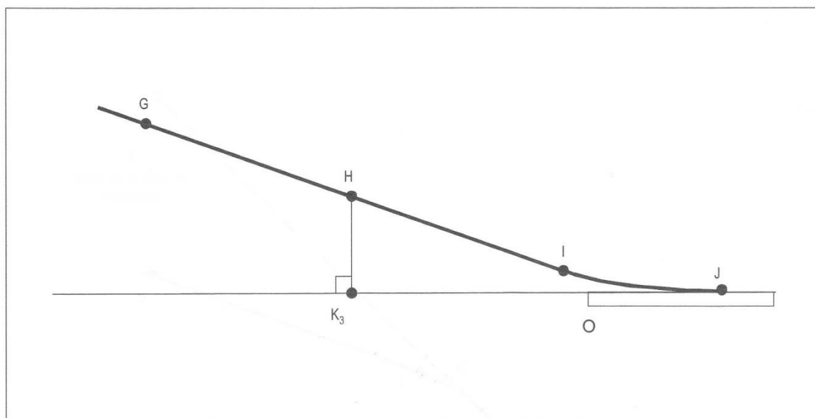
Rys. A2-6. Charakterystyki wzorcowego profilu dla podejścia do lądowania samolotu
