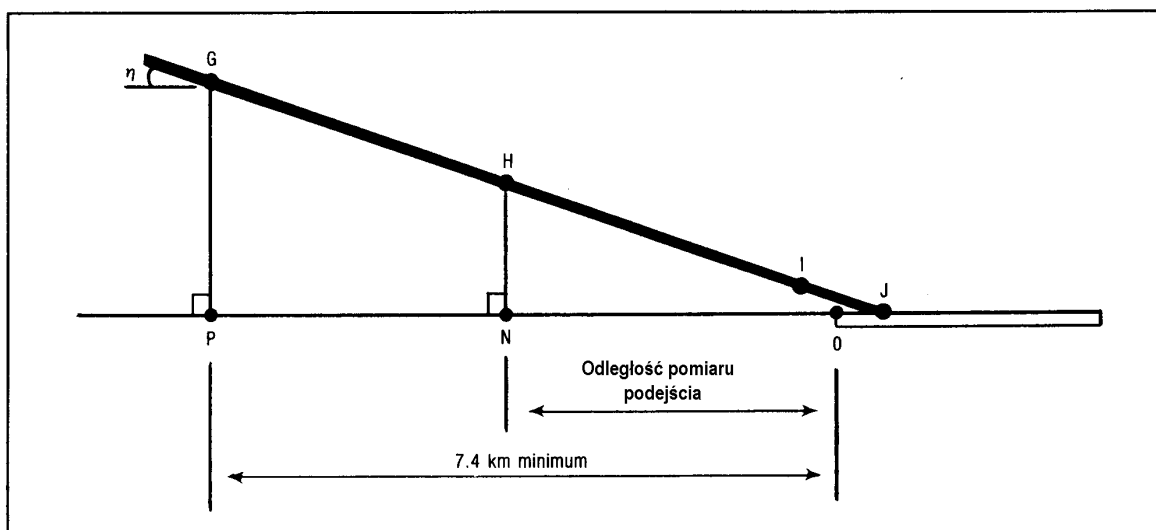
Rys. A1-7. Zmierzony profil podejścia
