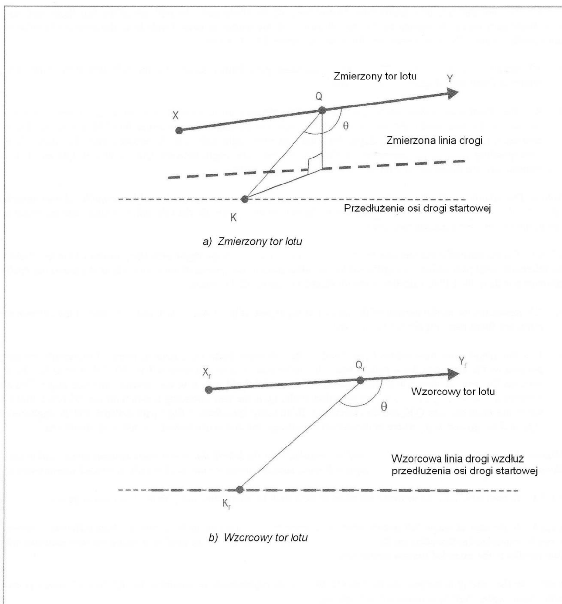
Rys. A2-10. Charakterystyki profilu wpływające na poziom hałasu dla mikrofonu umieszczonego pod torem lotu
