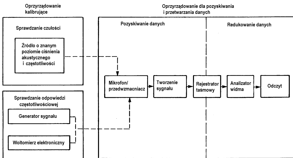
Rys. C-1. Układy pomiaru hałasu
