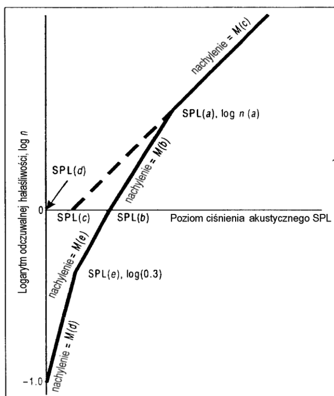
Rys. A2-3. Hałaśliwość odczuwalna w funkcji poziomu ciśnienia akustycznego.
