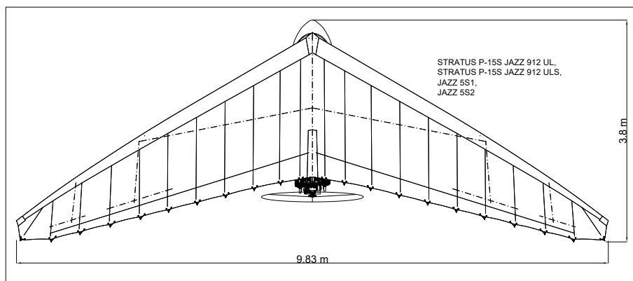
Rys. 1. Widok ogólny i podstawowe wymiary motolotni:
