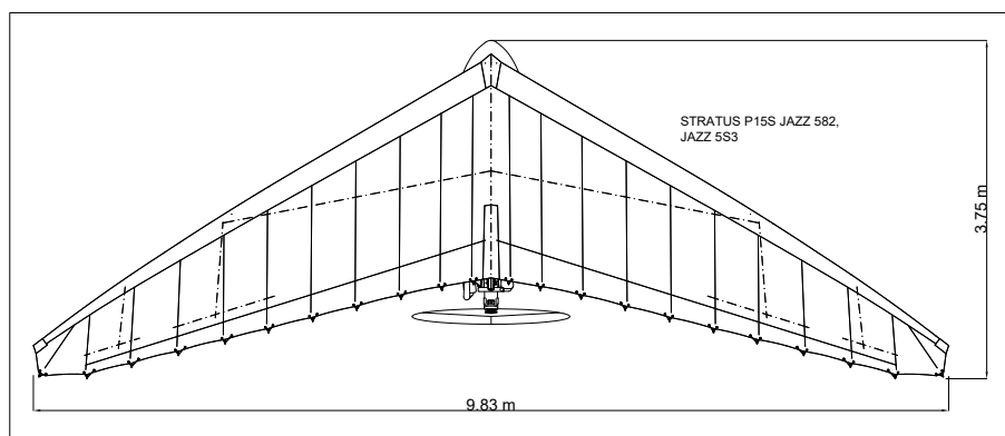
Rys. 2. Widok ogólny i podstawowe wymiary motolotni: STRATUS P-15S JAZZ 582, JAZZ 5S3
