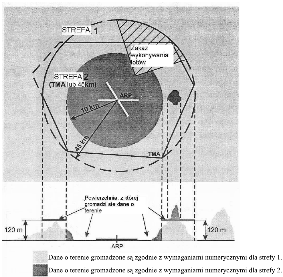
Rysunek A8-1. Powierzchnie, z których gromadzi się dane o terenie — strefa 1 i strefa 2.
