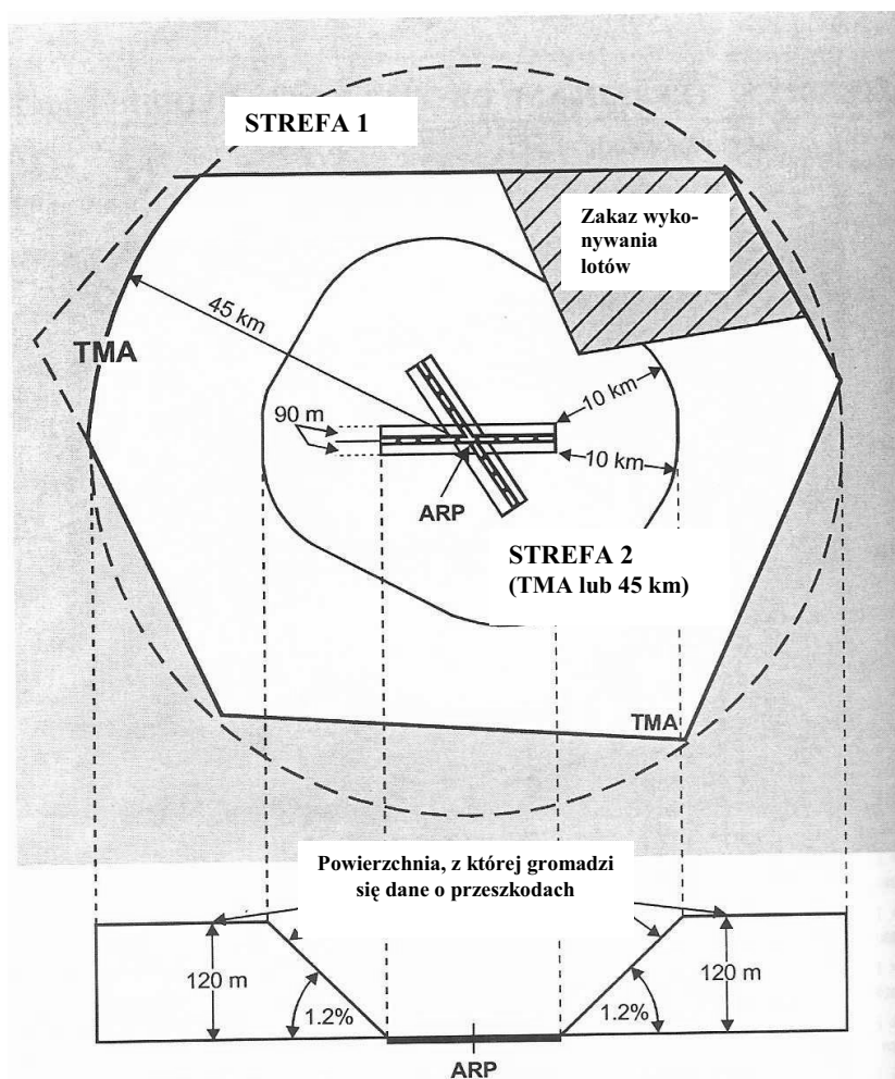
Rysunek A8-2. Powierzchnie, z których gromadzi się dane o przeszkodach — strefa 1 i strefa 2.
