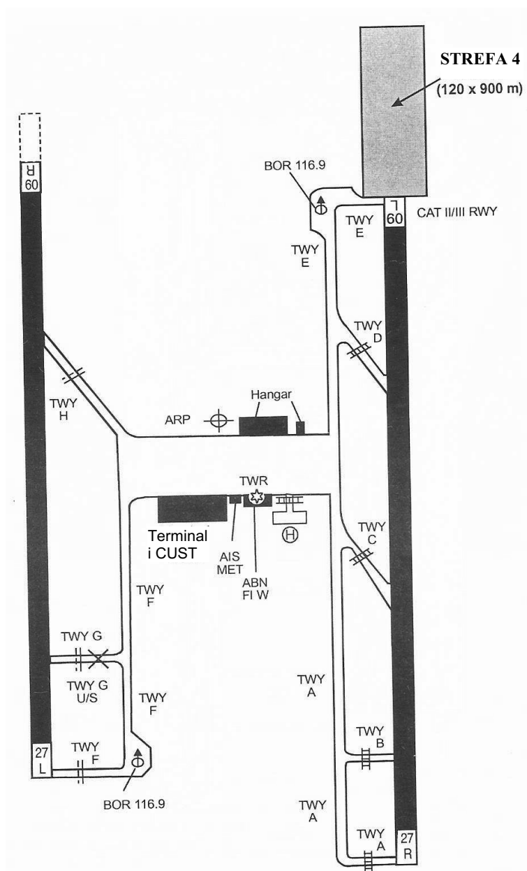
Rysunek A8-4. Powierzchnia, z której gromadzi się dane o terenie — strefa 4
