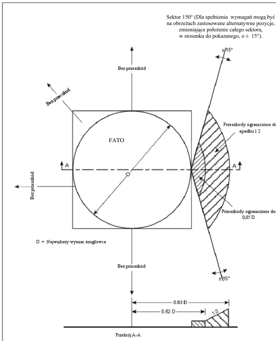
Rysunek 4-3. Sektory ograniczenia przeszkód na lotnisku dla śmigłowców na morzu. Śmigłowce jednowimikowe i dwuwimikowe w układzie poprzecznym.
