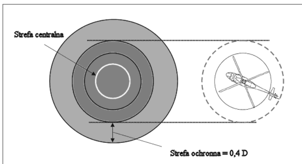
Rysunek 3-5. Obszar ochrony stanowiska postojowego śmigłowca
