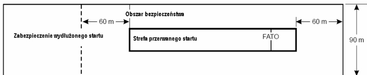
Rysunek 3-1. Obszar bezpieczeństwa dla FATO przyrządowego
