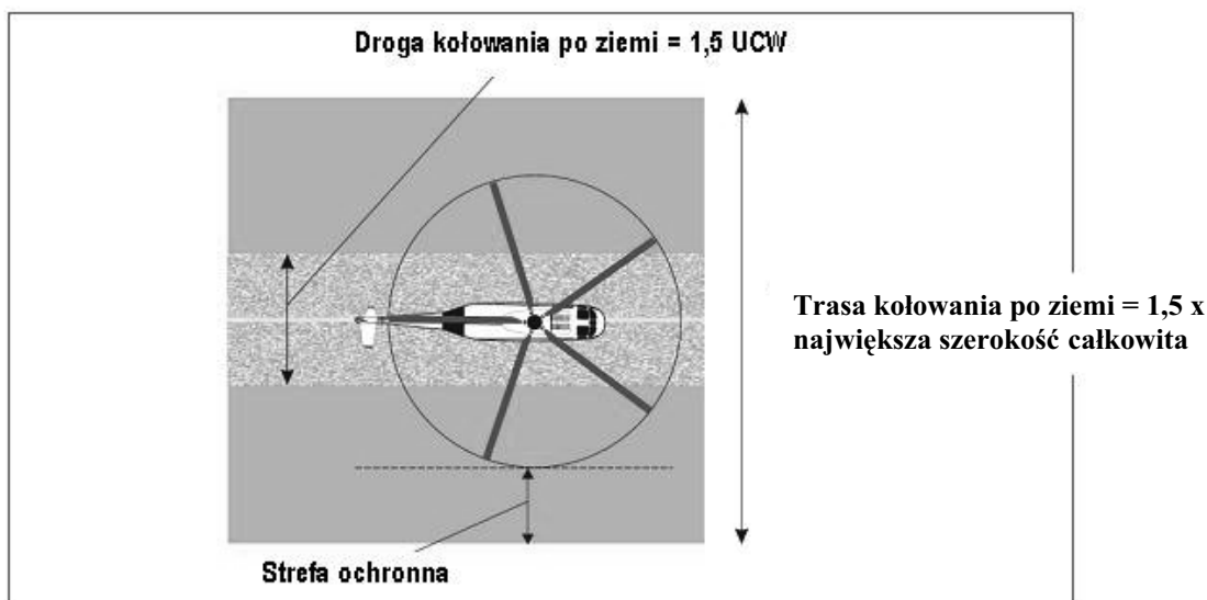
Rysunek 3-2. Trasa kołowania po ziemi
