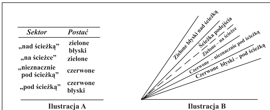
Rysunek 5-13. Światła postać sygnałów HAPI
