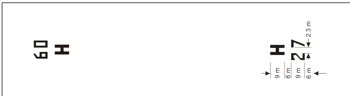
Rysunek 5-3. Oznakowanie identyfikacji strefy FATO oraz oznakowanie identyfikacji lotniska dla śmigłowców dla strefy FATO typu droga startowa
