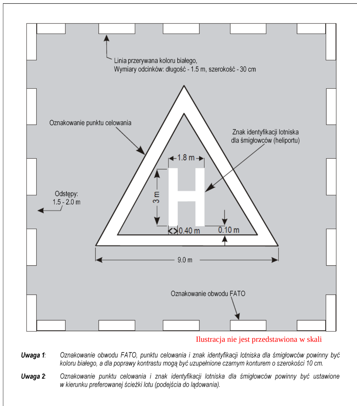
Rysunek 5-1. Połączone oznakowanie identyfikacji lotniska dla śmigłowców, oznakowanie punktu celowania i obwodu strefy FATO
