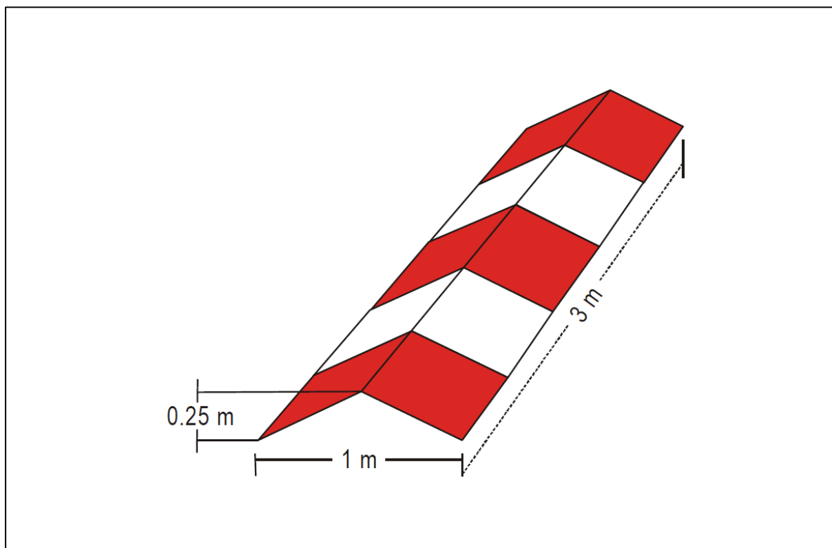
Rysunek 5-6 Oznacznik krawędzi strefy FATO typu droga startowa
