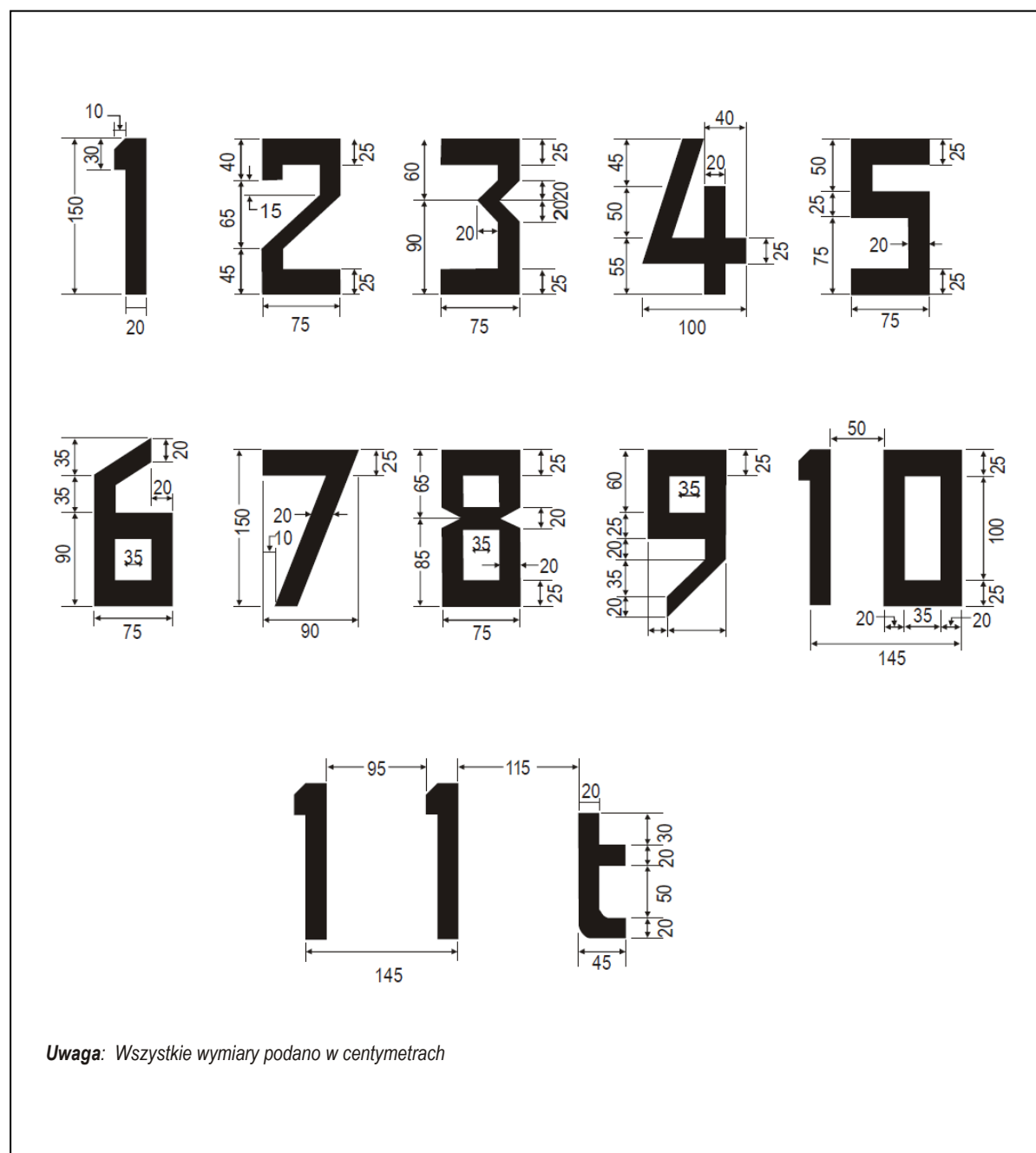
Rysunek 5-5 Kształt i proporcje liter i cyfr
