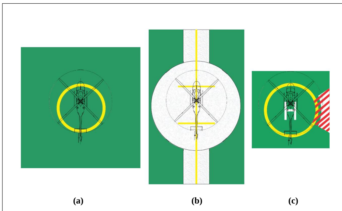
Rysunek 5-8. Oznakowanie przyziemienia / ustawienia pozycji (TDPM):
